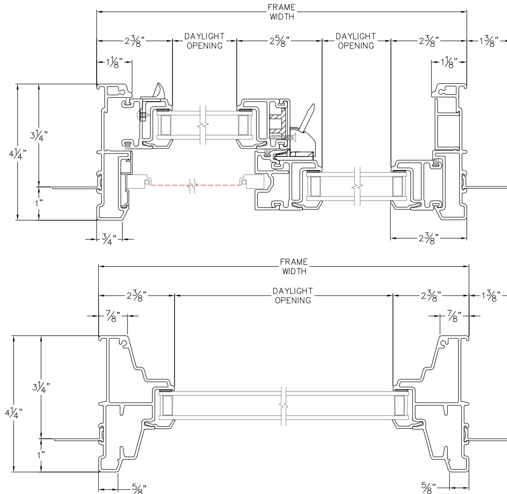
JAMBS
