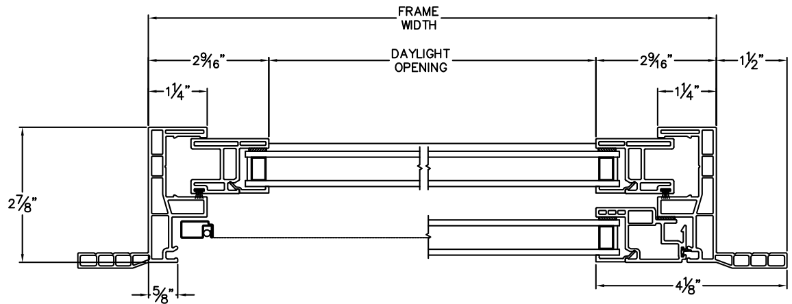
JAMBS
