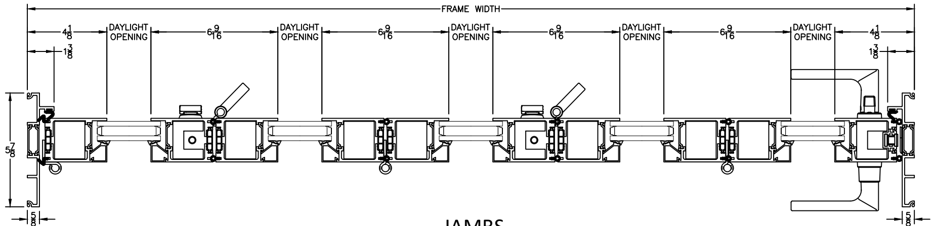
JAMBS
