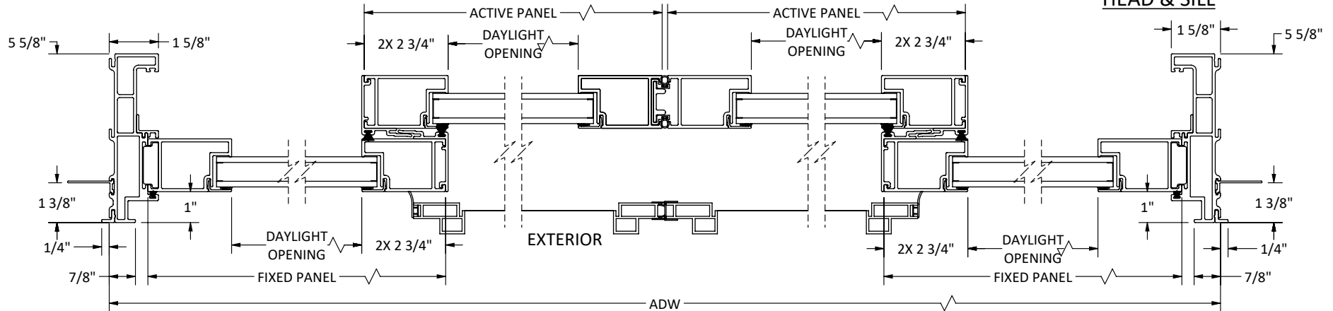
JAMBS
