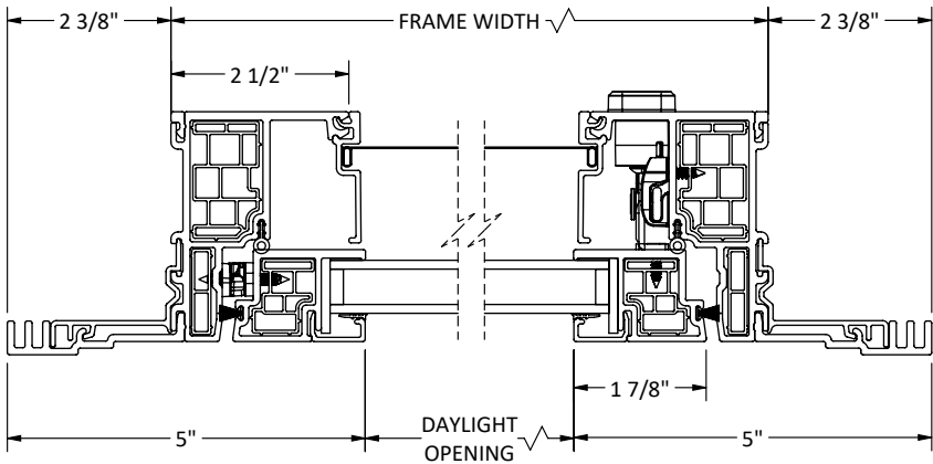
JAMBS
