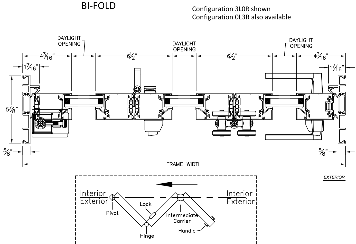
JAMBS
