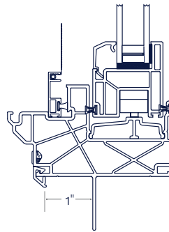
1" Mounting Fin Set-back
